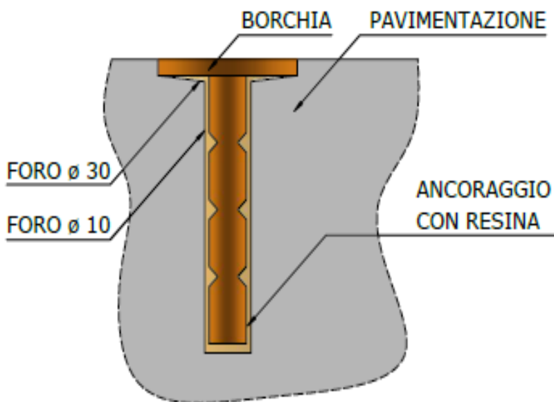
SEZIONE BORCHIA POSATA IN OPERA
