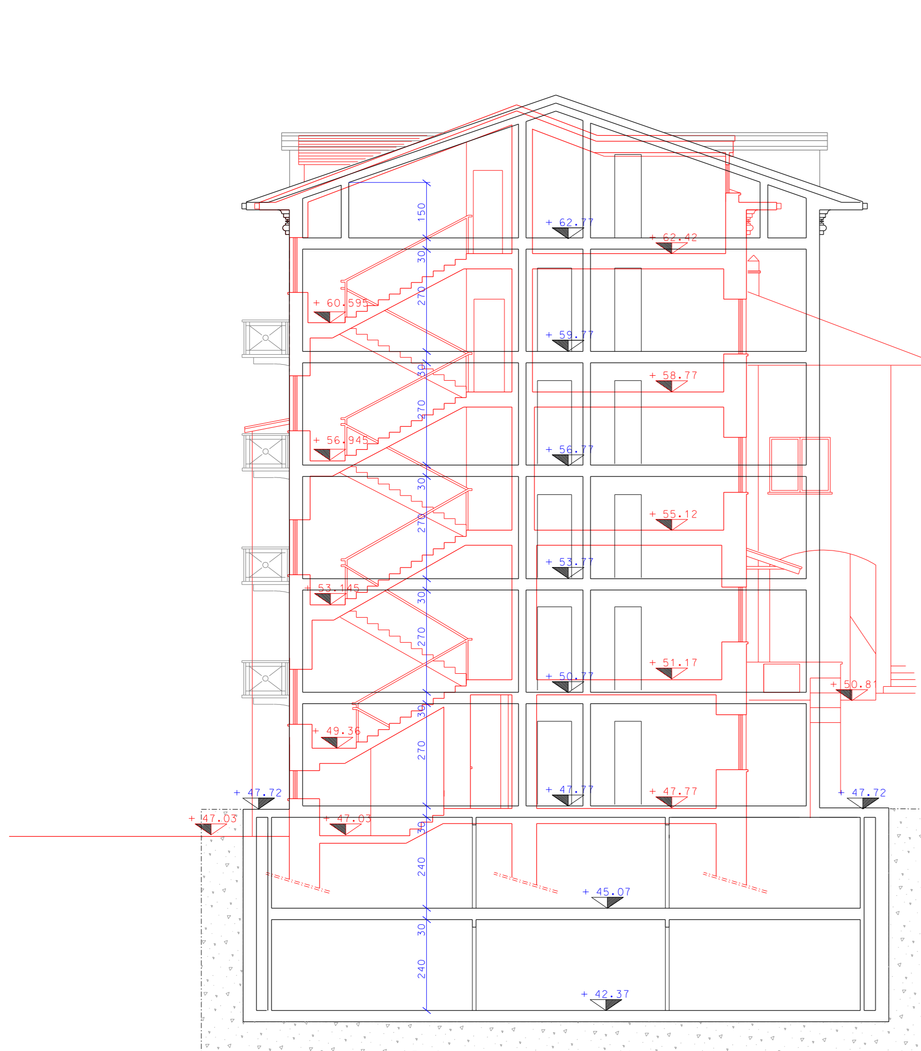
Sezione C C'
