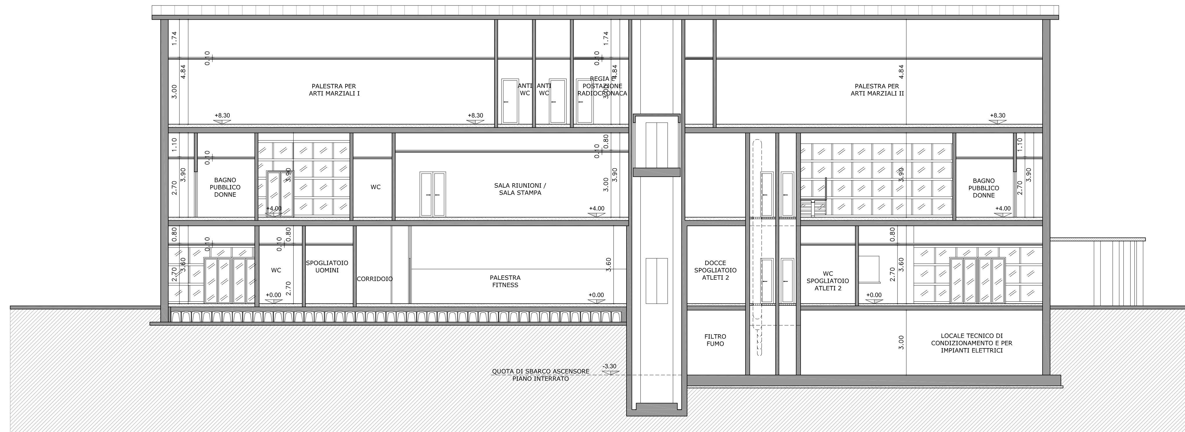
SEZIONE B-B' , SCALA 1:100
